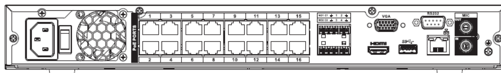
Figura 2-36 Panel trasero
