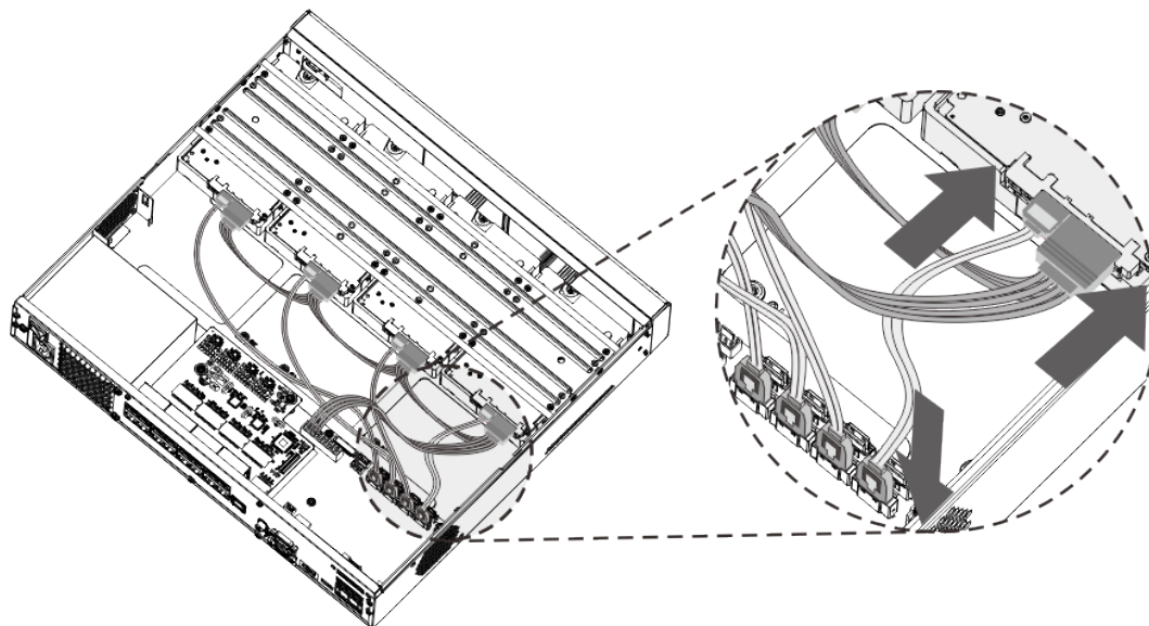
Figura 3-26 Cables de conexión
