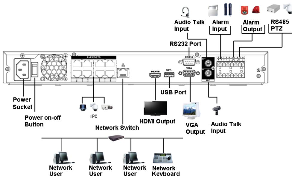
Figura 3-53 Conexión típica
