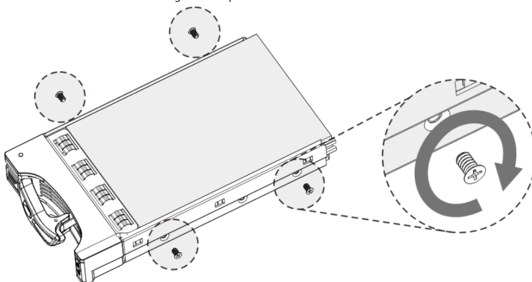
Figura 3-35 Apriete los tornillos
