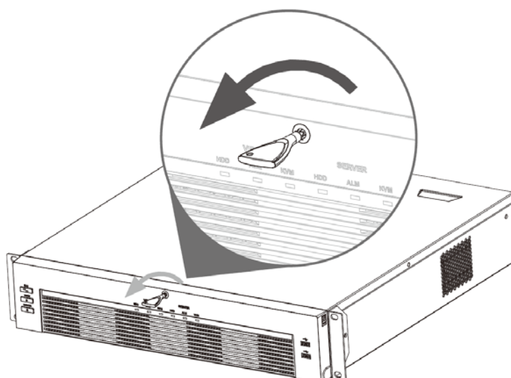
Figura 3-30 Fijar HDD
