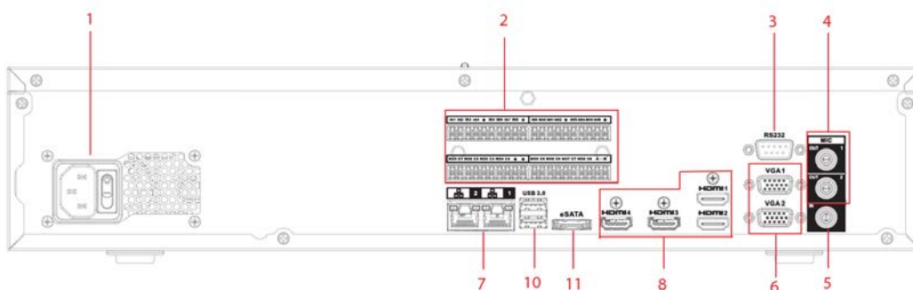
Figura 2-76 Panel trasero (3)
