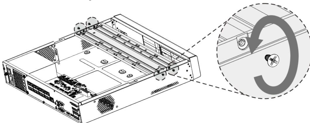
Figura 3-21 Retire los tornillos (2U)
