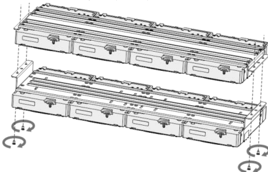
Figura 3-24 Soportes de bloqueo
