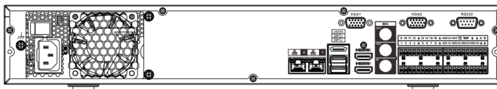
Figura 2-39 Panel trasero
