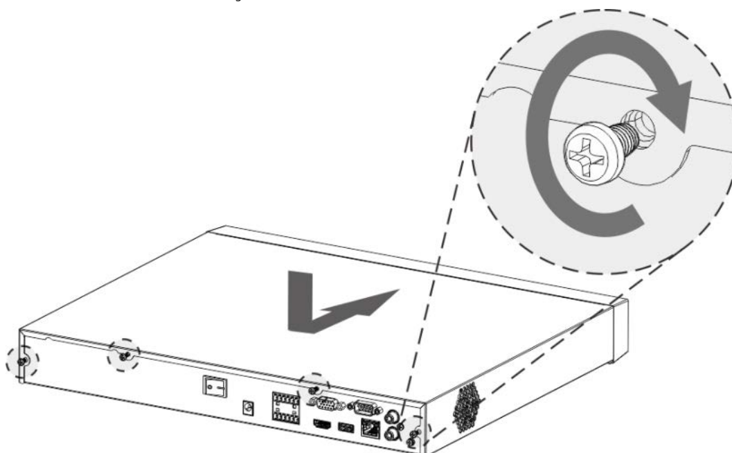
Figura 3-17 Vuelva a colocar la cubierta
