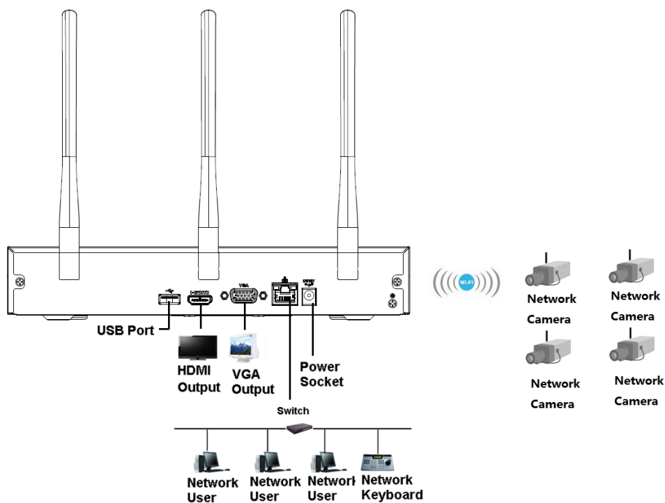
Figura 3-49 Conexión típica
