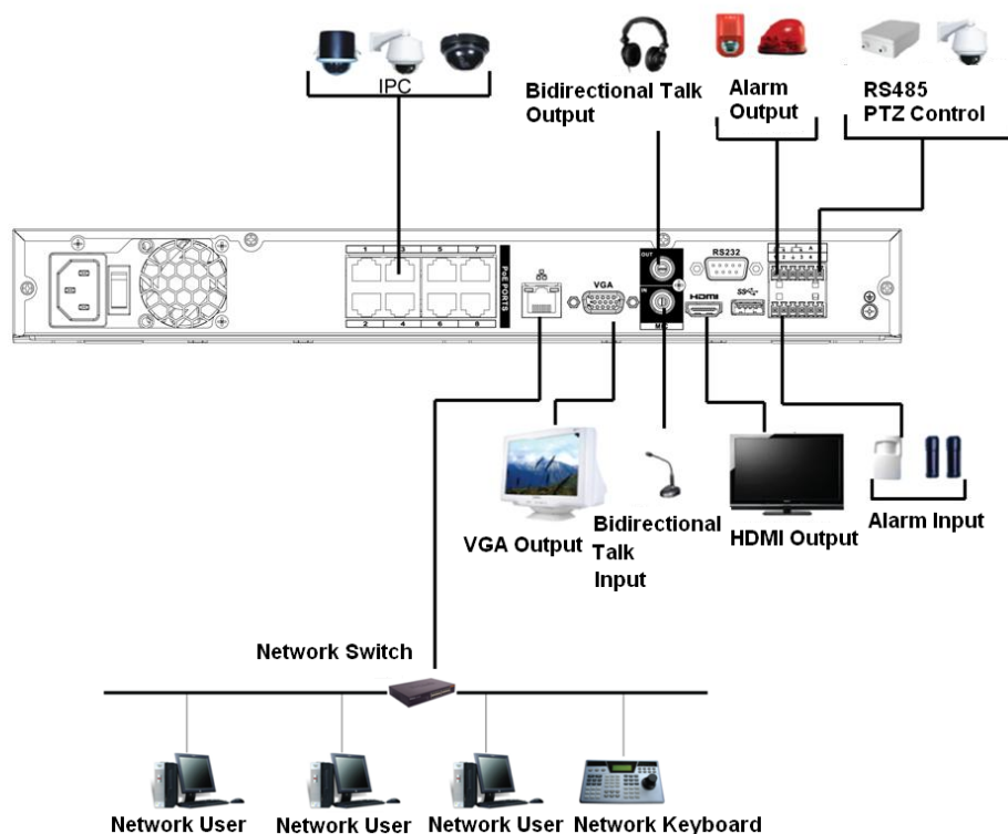
Figura 3-52 Conexión típica
