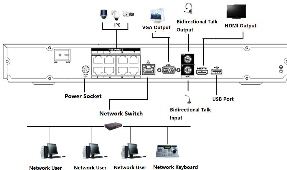
Figura 3-51 Conexión típica
