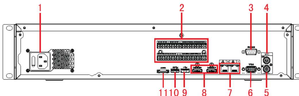
Figura 2-76 Panel trasero (3)
