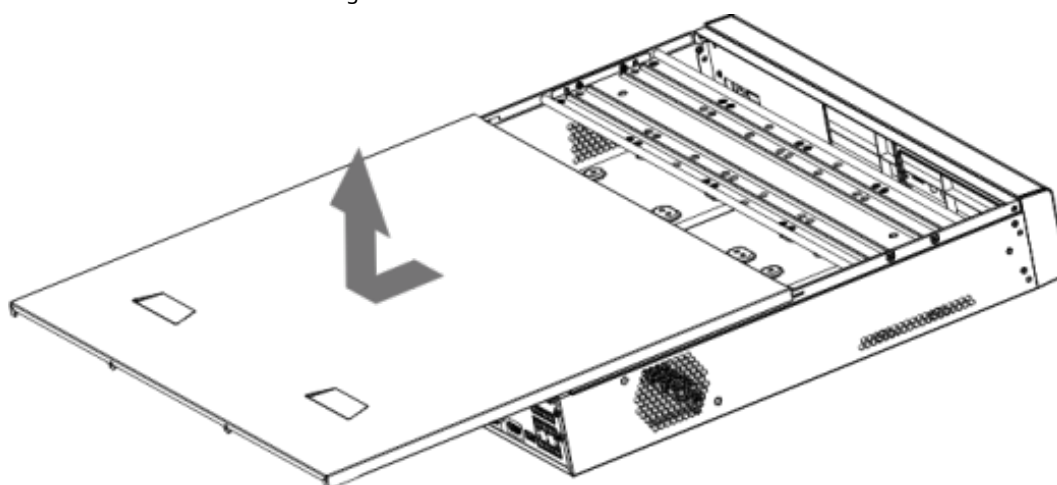
Figura 3-19 Retire la cubierta
