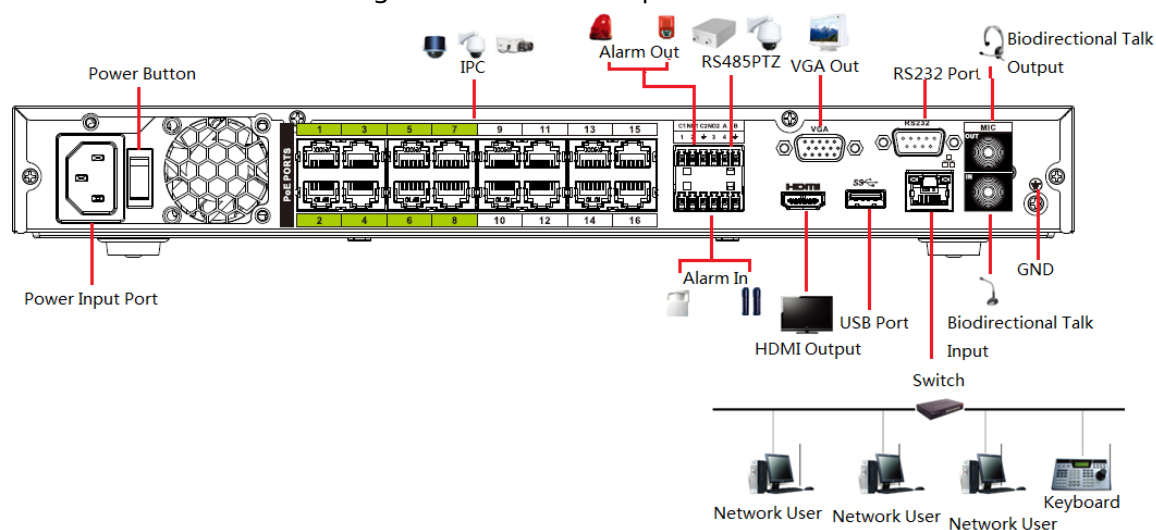
Figura 3-59 Conexión típica
