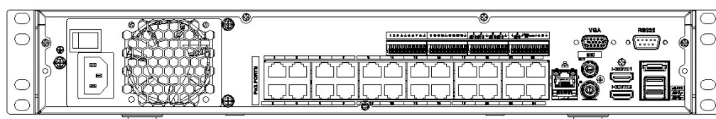
Figura 2-41 Panel trasero
