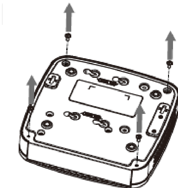
Figura 3-2 Tornillos sueltos
