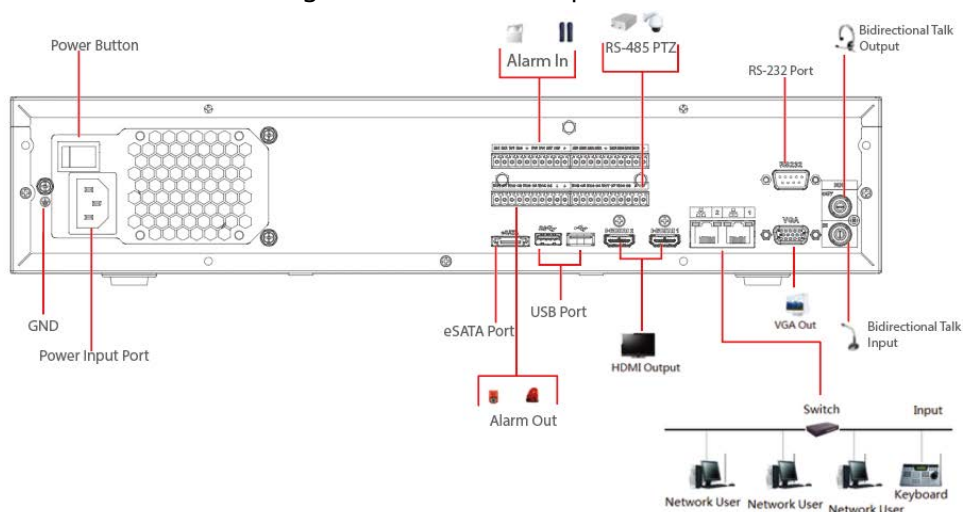
Figura 3-61 Conexión típica
