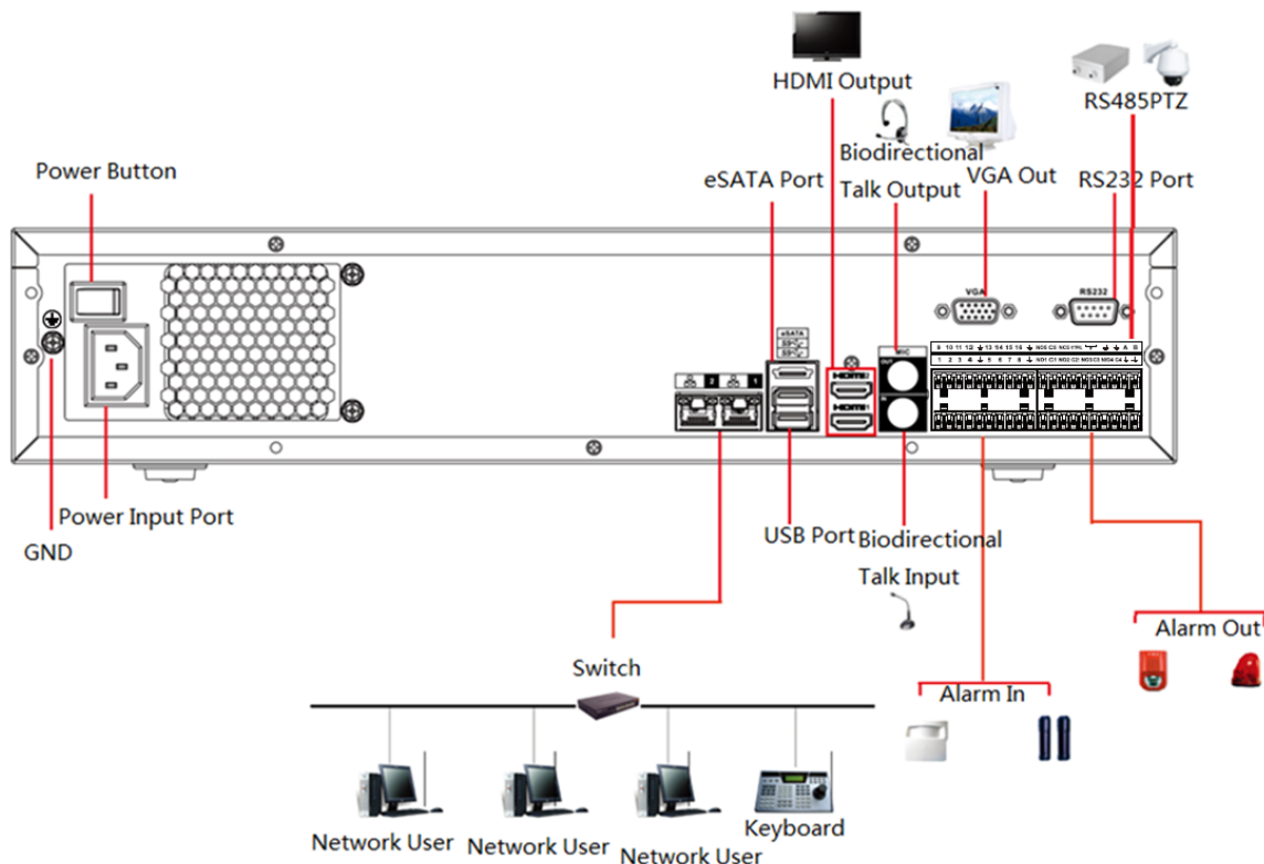
Figura 3-57 Conexión típica
