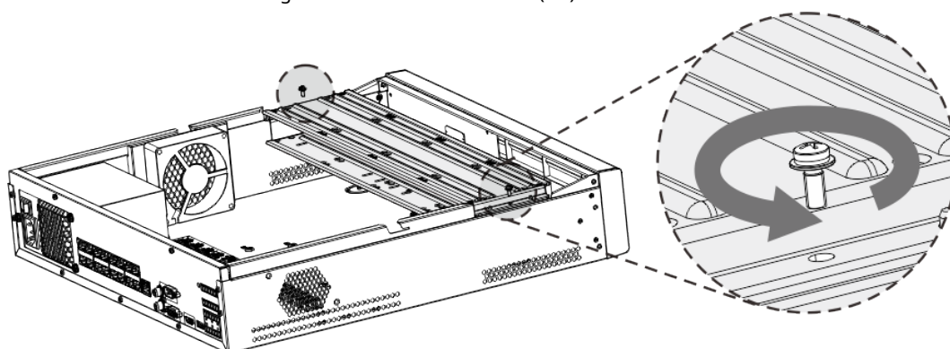
Figura 3-21 Retire los tornillos (2U)
