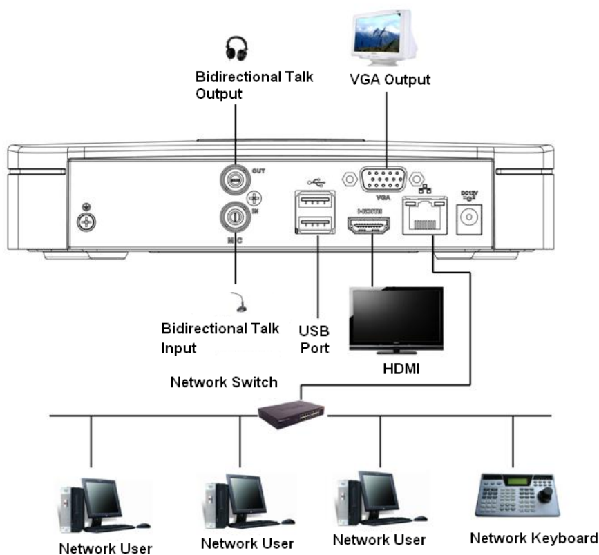
Figura 3-48 Conexión típica
