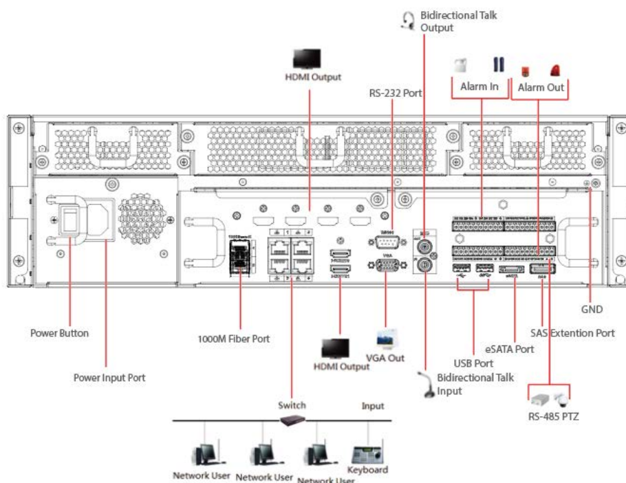
Figura 3-62 Conexión típica
