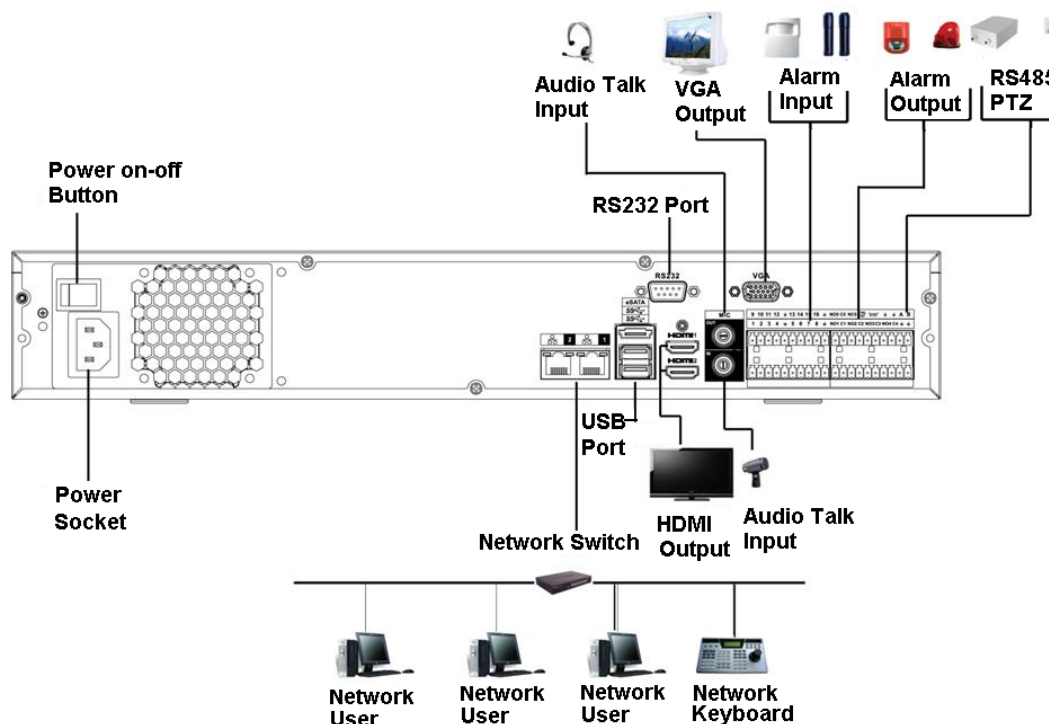
Figura 3-54 Conexión típica
