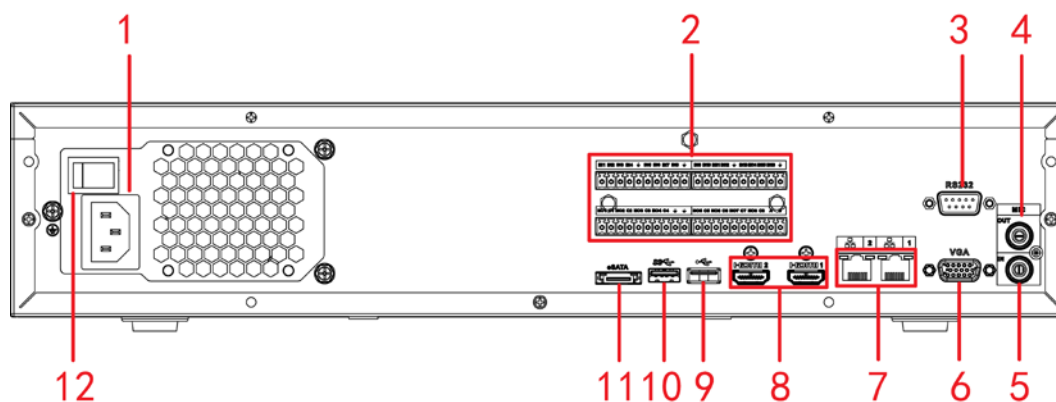
Figura 2-74 Panel trasero (1)
