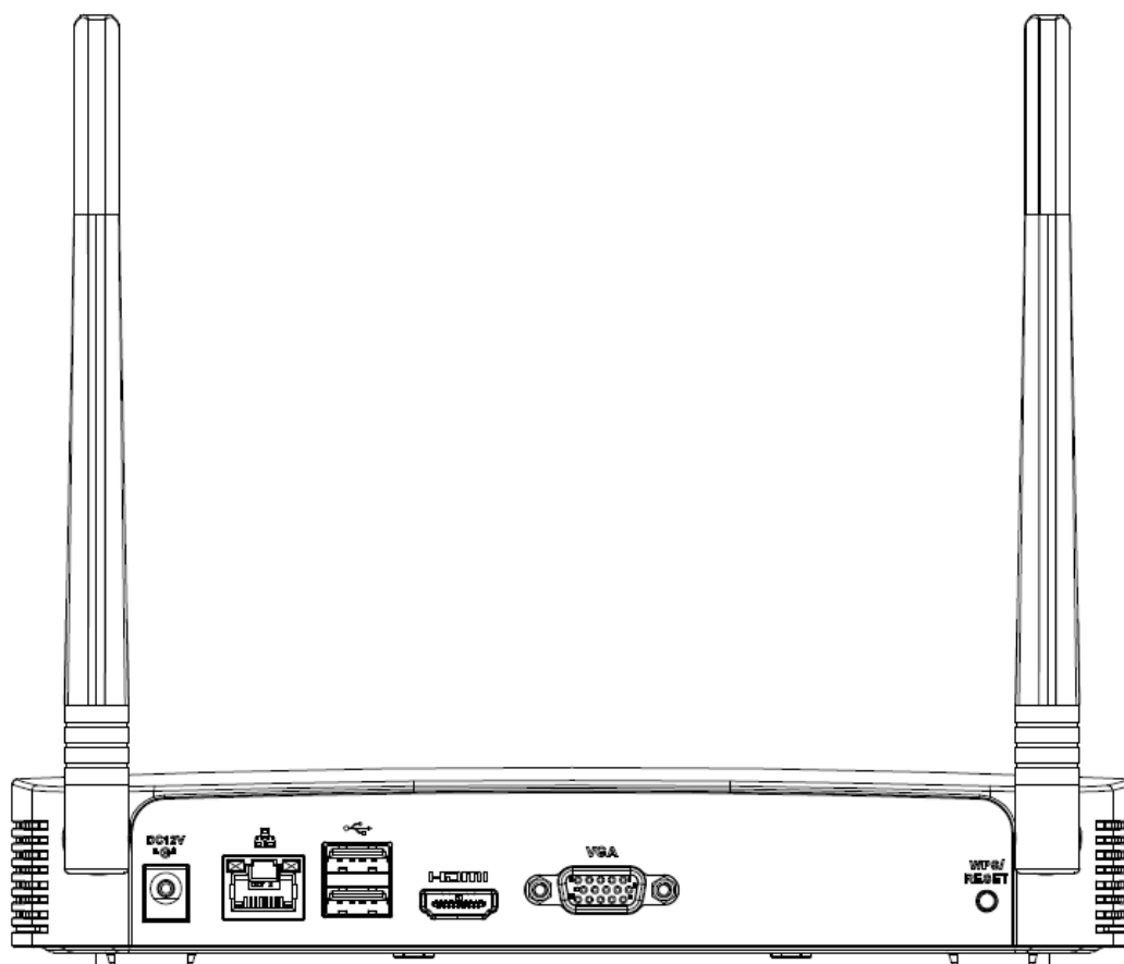
Figura 2-55 Panel trasero
