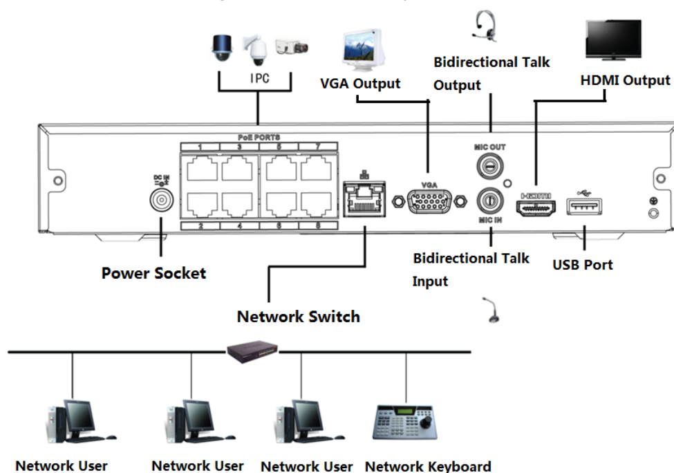
Figura 3-50 Conexión típica
