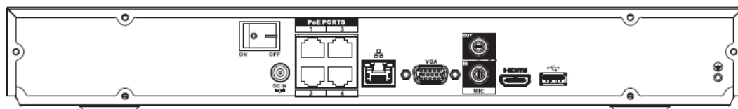
Figura 2-32 Panel trasero
