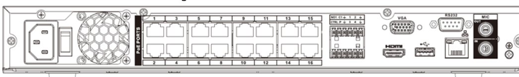
Figura 2-50 Panel trasero
