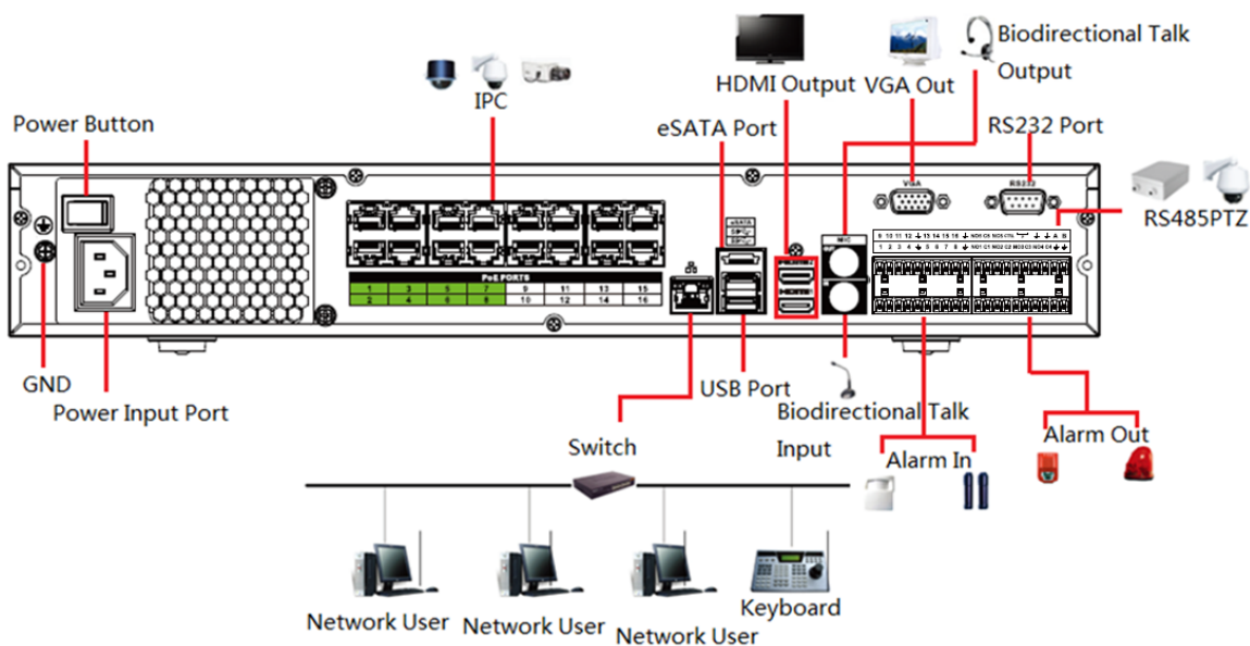
Figura 3-58 Conexión típica
