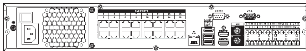
Figura 2-40 Panel trasero
