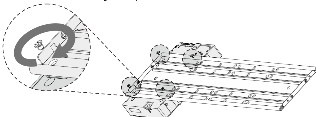
Figura 3-22 Apriete los tornillos
