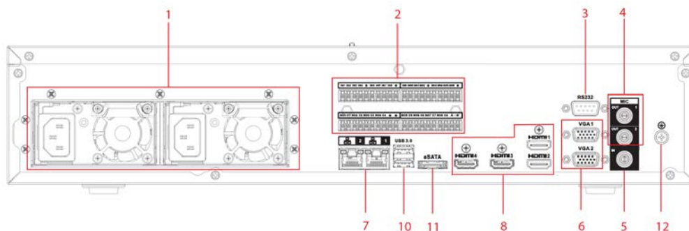
Figura 2-77 Panel trasero (4)
