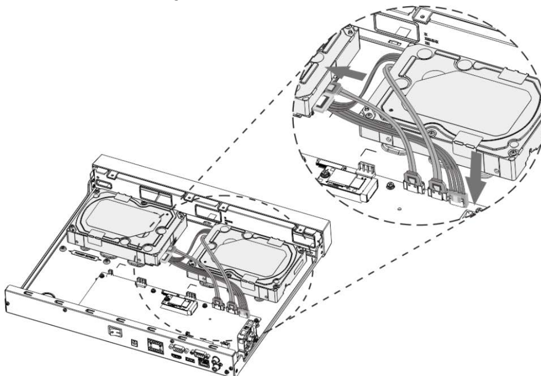
Figura 3-16 Cables de conexión
