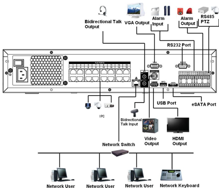
Figura 3-56 Conexión típica
