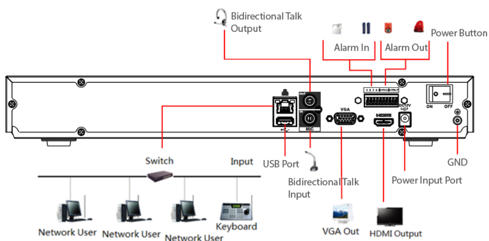
Figura 3-60 Conexión típica
