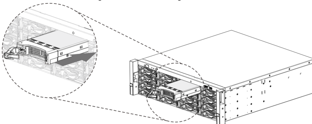
Figura 3-36 Cerrar el mango
