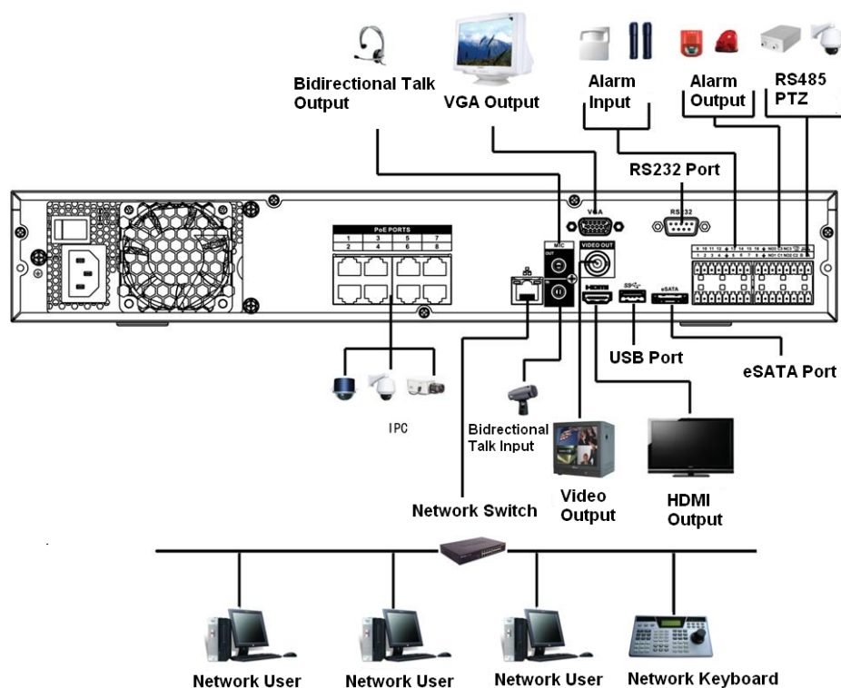
Figura 3-55 Conexión típica
