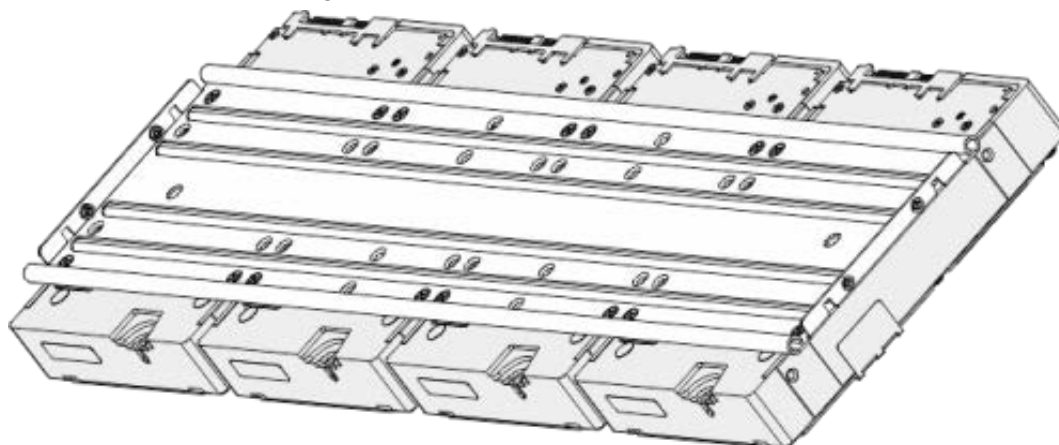
Figura 3-23 Instale más discos duros
