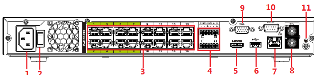
Figura 2-71 Panel trasero
